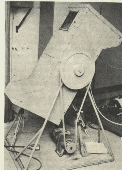
Bindningsmetoderna provades i denna falltrumma hos Statens provningsanstalt.
